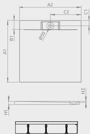
zuhanytálca lábbal
